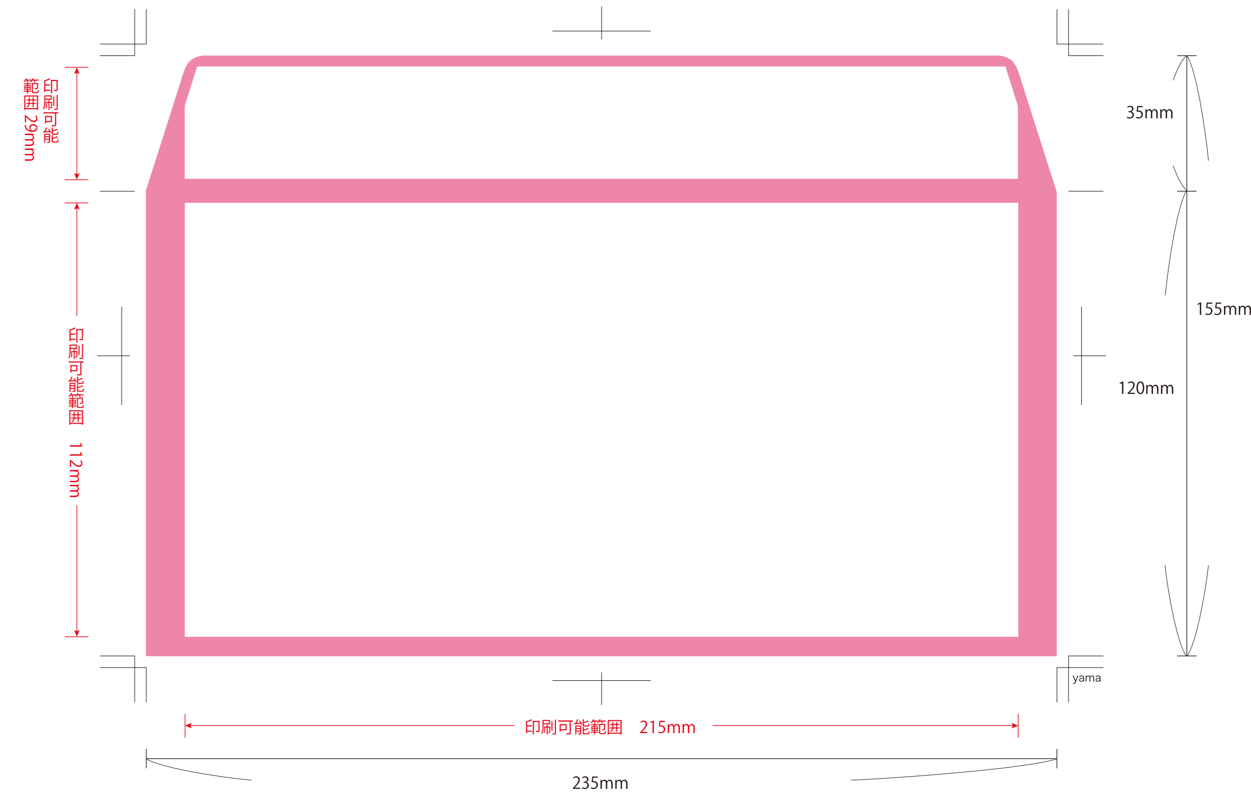
洋長3カマス天タテ_テンプレート_表
